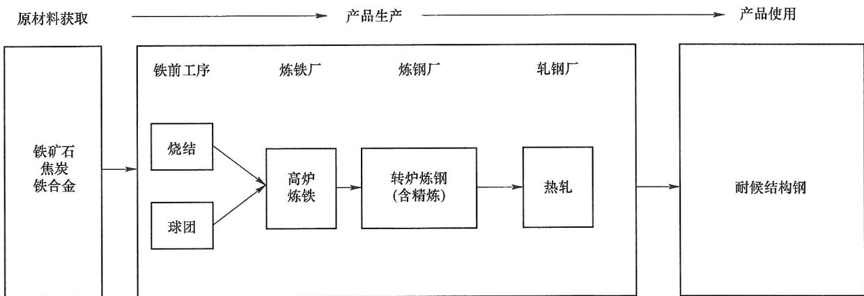
图 A.1 耐候结构钢生命周期系统边界示意图
